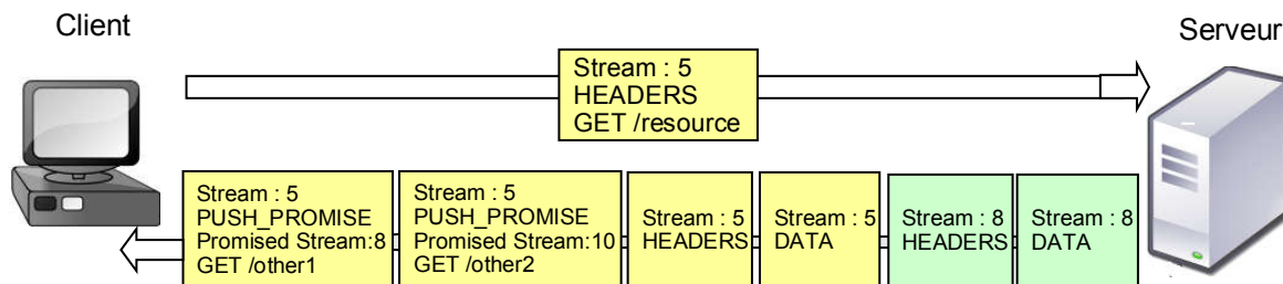
Figure 5 : Mécanisme de « server push »
