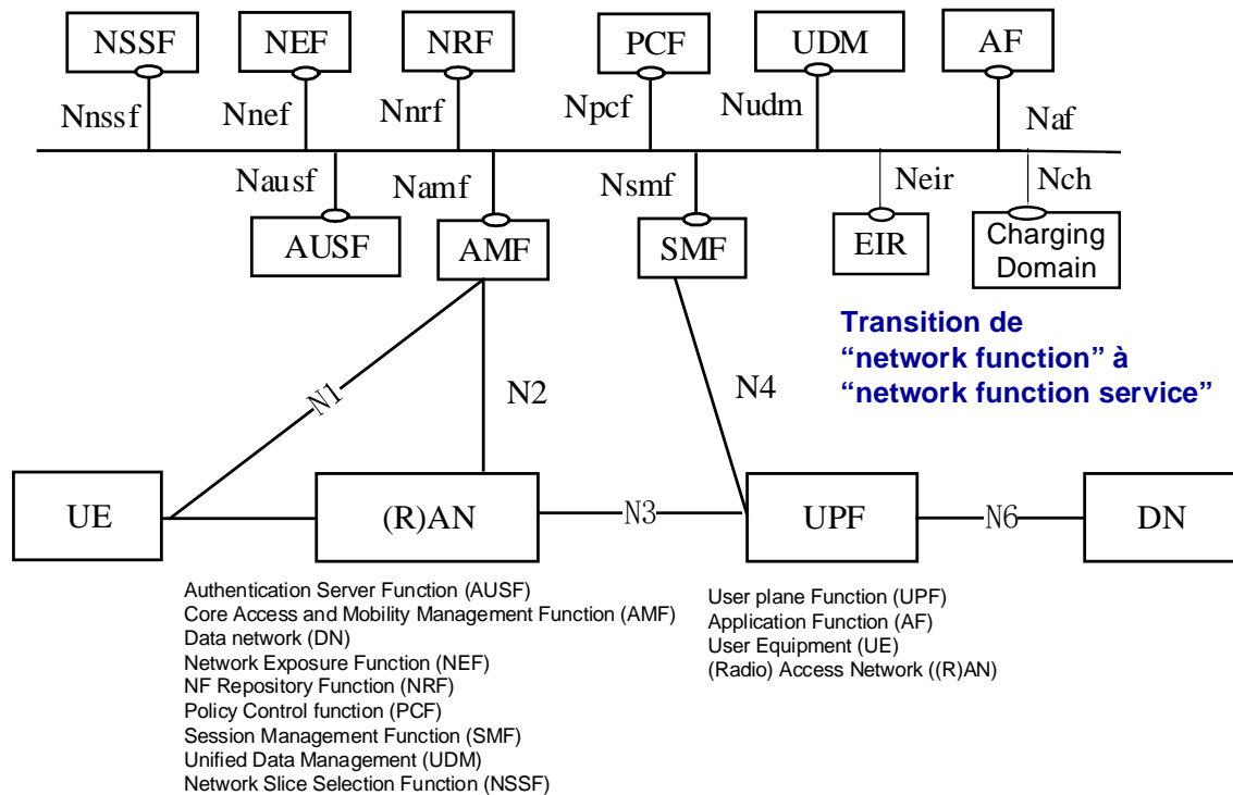
Figure 6 : Fonctions réseau 5GC et leur interface de service
