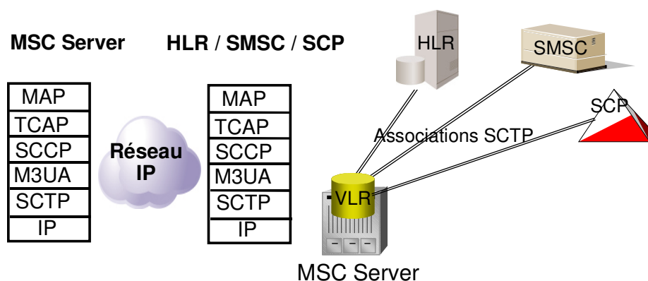
Figure 10 : M3UA en mode symétrique
