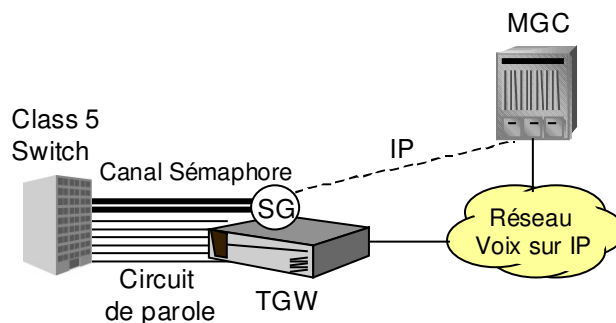
Figure 5 : Scénario d'usage M2UA dans le contexte NGN Fixe
