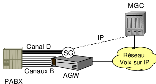
Figure 3: Scénario d'usage IUA
