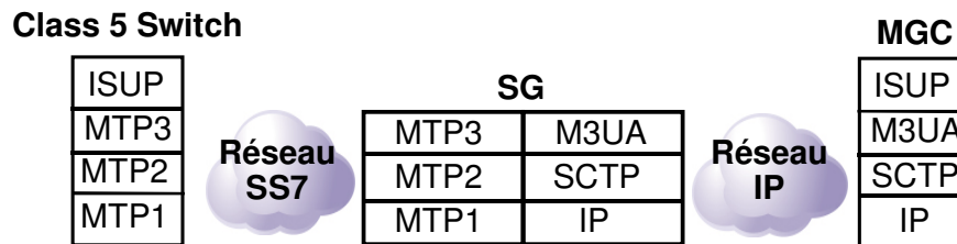
Figure 9 : Transport de la signalisation ISUP/MTP3 par M3UA
