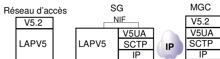
Figure 8 : Transport de la signalisation V5.2 par V5UA
