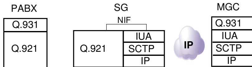
Figure 4 : Transport de la signalisation Q.931 par IUA
