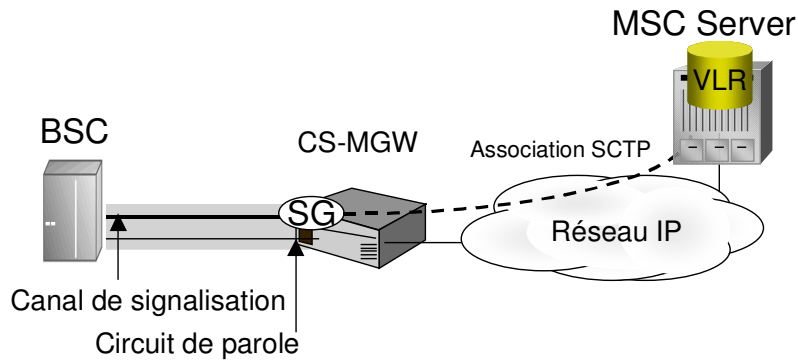
Figure 7 : Scénario d'usage M2UA dans le contexte NGN Mobile
