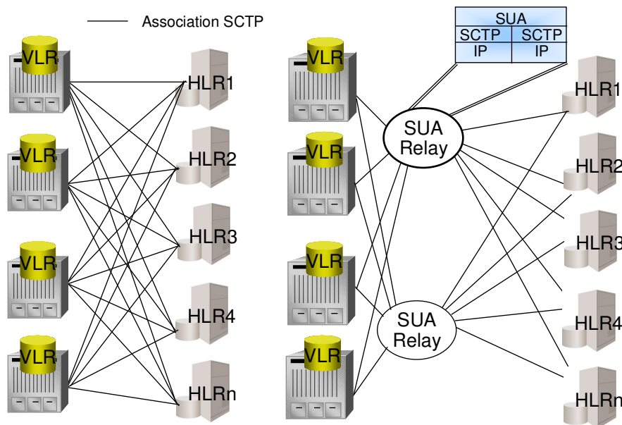
Figure 14 : Utilisation de l'entité SUA Relay
