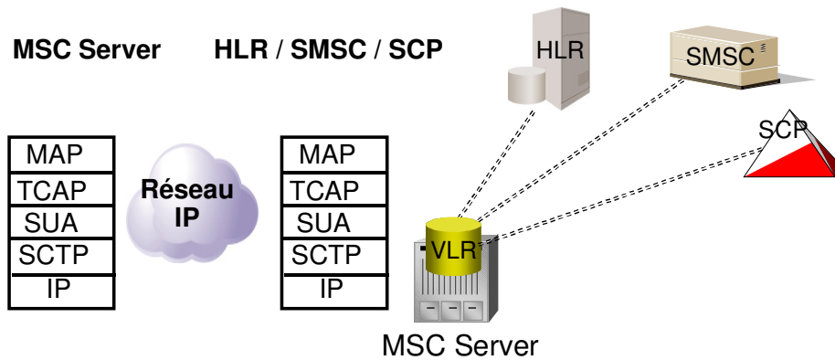
Figure 13 : Scénario d'usage SUA en mode symétrique dans le contexte NGN Mobile
