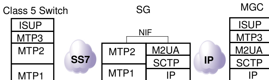
Figure 6 : Transport de la signalisation ISUP/MTP3 par M2UA
